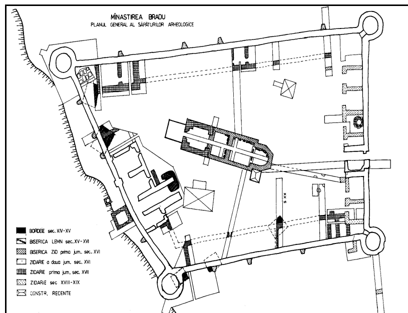
Fig. 7. Bradu, jud. Buzău. Planul mănăstirii, după Ion Chicideanu și Constanța Modoran, 1983.
