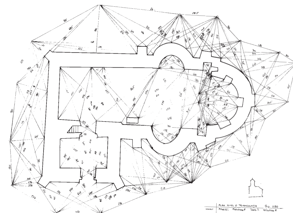
Fig. 3 Planul bisericii
